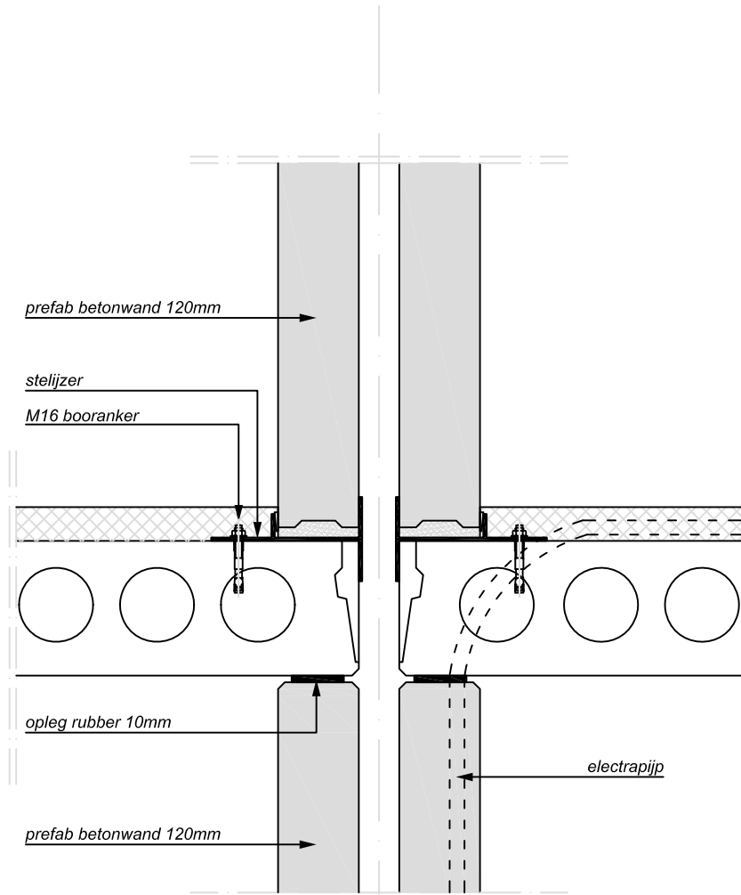
Detail Casco bouw schaal 1:10
