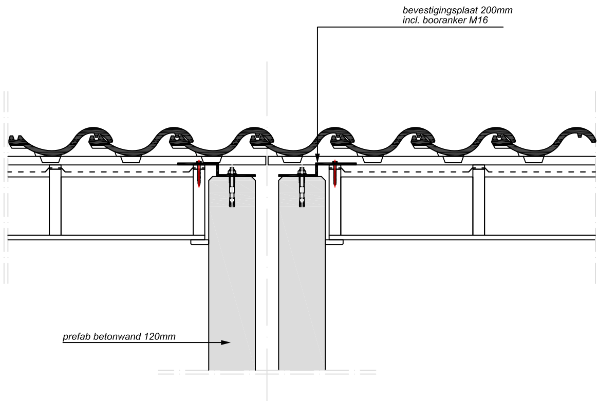
Detail Casco bouw schaal 1:10
