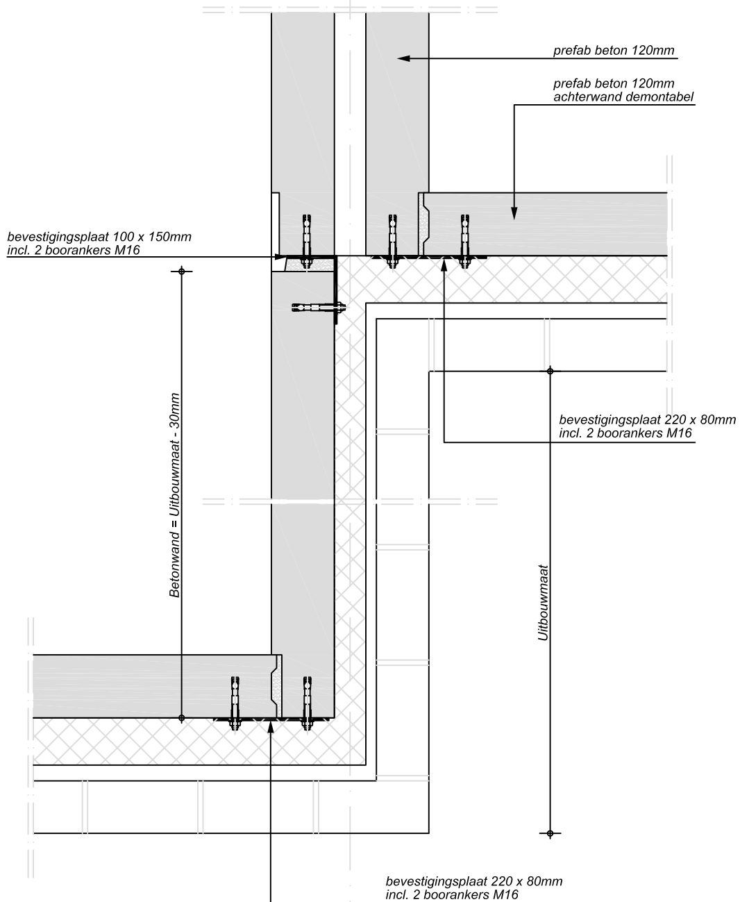
Detail Casco bouw schaal 1:10
