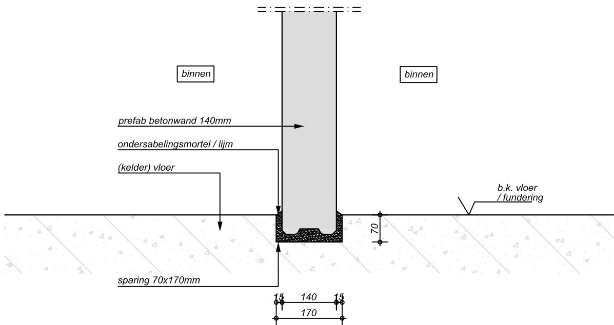
Detail mestkelder wand schaal 1:10
